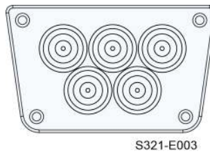
figure 5-3 Plaque d'étanchéité CA de rechange
